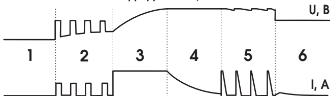
ЭТАПЫ ЗАРЯДА ДЛЯ WET, AGM/GEL АКБ
