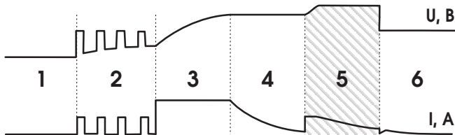
ЭТАПЫ ЗАРЯДА ДЛЯ Ca/Ca АКБ
