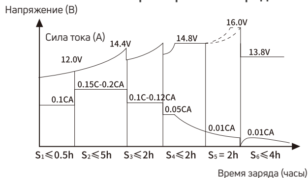
Характеристики заряда
